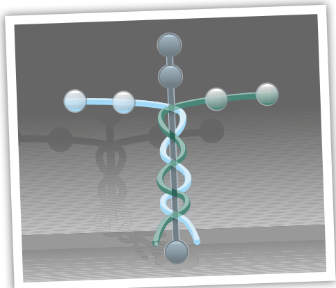
Laminin
